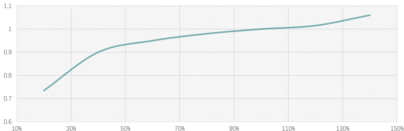
连接导线截面/标准截面
